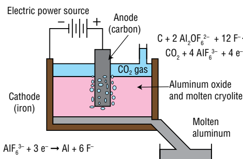
La figura 2. La electrólisis del óxido de aluminio
