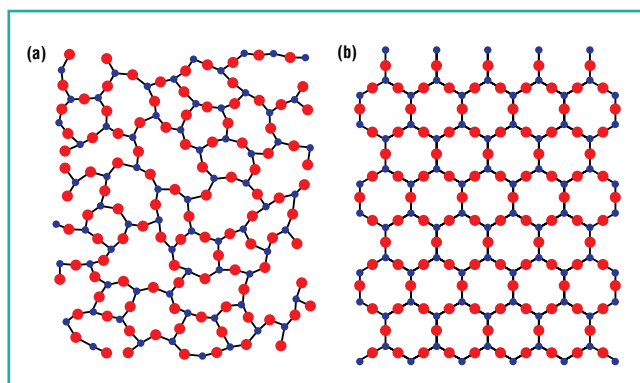
Figura 1. Comparación de las estructuras químicas de (a) un sólido amorfo hecha de dióxido de silicio (vidrio) y (b) un cristal de dióxido de silicio (cerámica)
